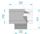
Дефлектор з нержавіючої сталі товщиною 1,0мм
