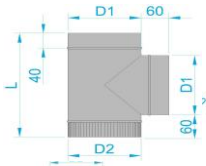
Трійник з нержавіючої сталі товщиною 1,0мм
