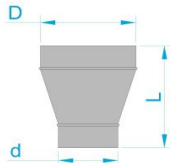
Прехідник з нержавіючої сталі товщиною 1,0мм
