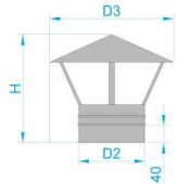
Дашок з нержавіючої сталі товщиною 1,0мм
