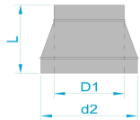
Закінчення димоходу (вн. товщиною 0,8мм/ зовн. товщиною 0,5мм )
