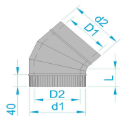
Коліно (вн. товщиною 0,5мм/ зовн. товщиною 0,5мм )
