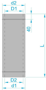
Труба (вн. товщиною 0,5мм/ зовн. товщиною 0,5мм )
