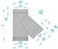
Трійник (вн. товщиною 0,5мм/ зовн. товщиною 0,5мм )
