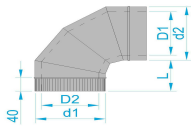
Коліно (вн. товщиною 0,8мм/ зовн. товщиною 0,5мм )
