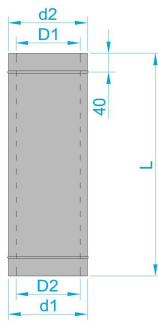
Труба (вн. товщиною 0,5мм/ зовн. товщиною 0,5мм )
