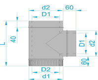
Трійник (вн. товщиною 0,8мм/ зовн. товщиною 0,5мм )
