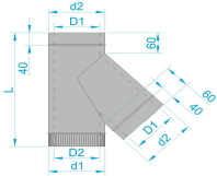
Трійник (вн. товщиною 0,5мм/ зовн. товщиною 0,5мм )
