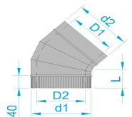
Коліно (вн. товщиною 0,5мм/ зовн. товщиною 0,5мм )
